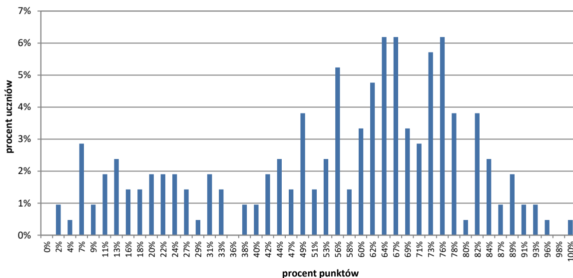
WYKRES 8. ROZKŁAD WYNIKÓW UCZNIÓW (ARKUSZ OPOP-C00-2405)
