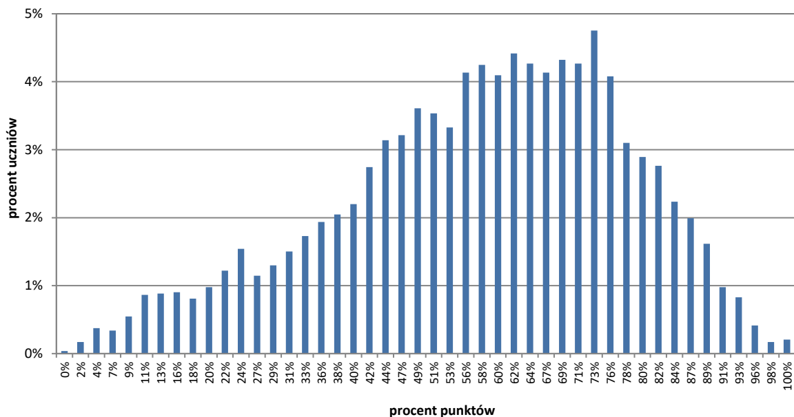
WYKRES 1. ROZKŁAD WYNIKÓW UCZNIÓW (ARKUSZ OPOP-100-2405)
