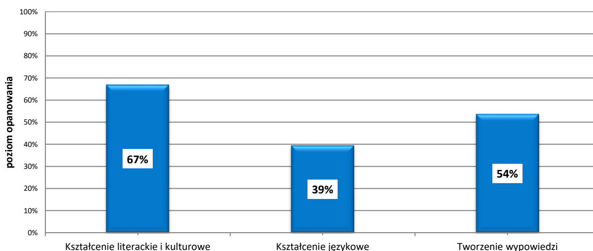
WYKRES 4. ŚREDNIE WYNIKI UCZNIÓW W ZAKRESIE POSZCZEGÓLNYCH OBSZARÓW UMIEJĘTNOŚCI (ARKUSZ OPOP-100-2405)
